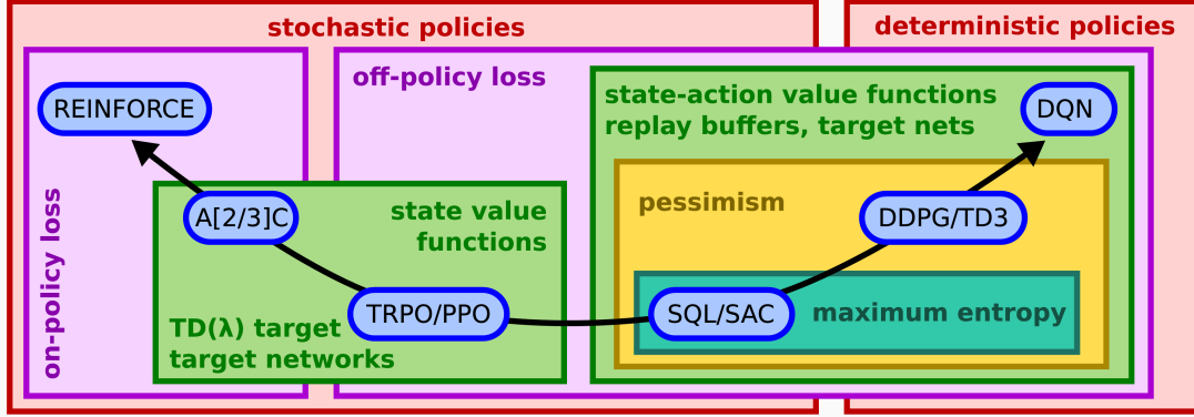
Figure 3: 策略梯度类算法谱图（来自 TU Delft 课件）
