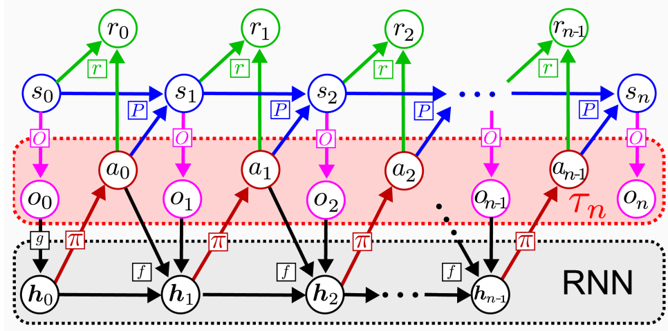
Figure 2: 部分可观马尔可夫链及 RNN 历史编码示意图（来自 TU Delft 课件）
