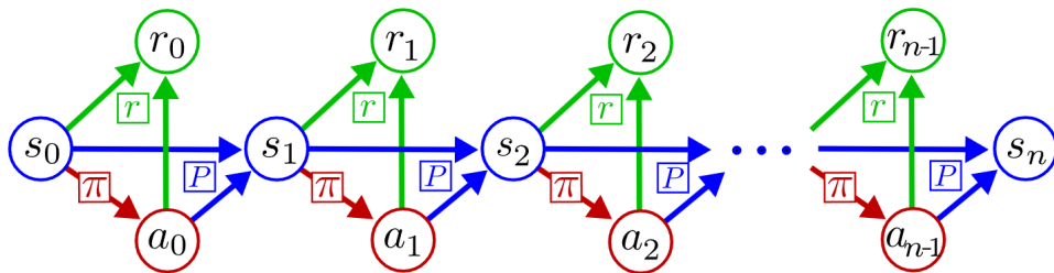
Figure 1: 马尔可夫链示意图（来自 TU Delft 课件）
